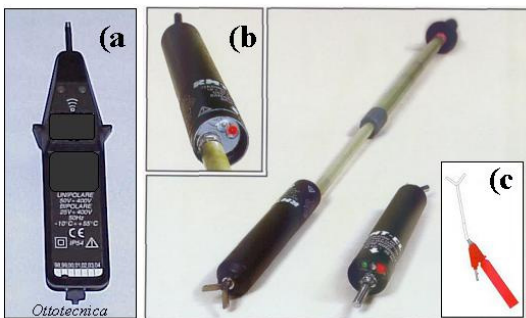
Fig. 11 Rivelatori di presenza/assenza di tensione: (a) per impianti BT, (b) per impianti MT da interno e (c) per impianti MT da esterno.
